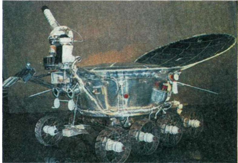
Рис. 7.11. «Луноход-1»
