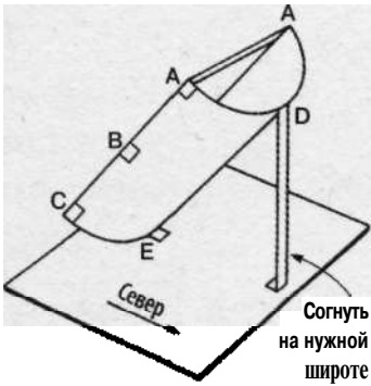
Рис. Л.2.2. Готовые солнечные часы
