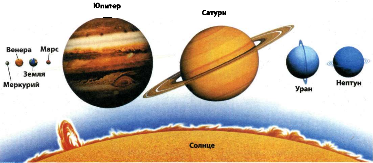
Рис. 1.12. Относительные размеры Солнца и планет Солнечной системы. Средний радиус Земли 6370 км
