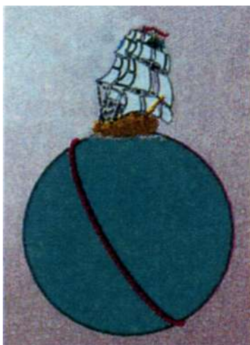
Рис. 15.11. Сфера может быть моделью двумерного безграничного мира, который имеет конечную площадь. В таком пространстве тоже можно совершить кругосветное путешествие — так Магеллан доказал, что поверхность Земли не имеет предела
