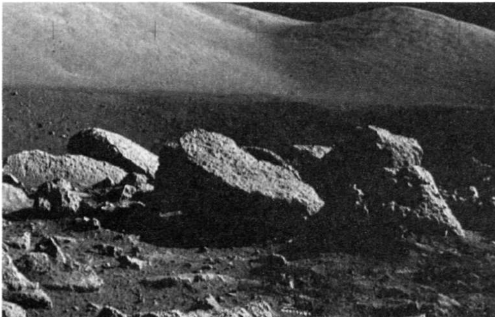
Рис. 7.12. Типичный лунный пейзаж. На поверхности преобладает темно-серый цвет грунта, припорошенный слоем реголита
