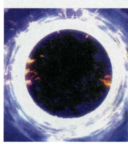
Рис. 14.9. Черная дыра
