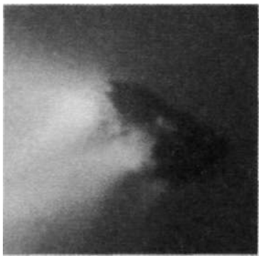
Рис. 11.10. Ядро кометы Галлея на расстоянии нескольких тысяч километров. Длина очень темного ядра 15 км, ширина — 8 км. Из отверстий, находящихся на поверхности, вырываются струи газа
