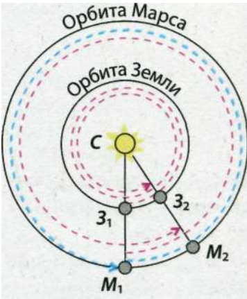
Рис. 4.2. Путь, соответствующий сидерическому периоду обращения Марса вокруг Солнца, изображен пунктиром синего цвета, синодическому — пунктиром красного цвета.
