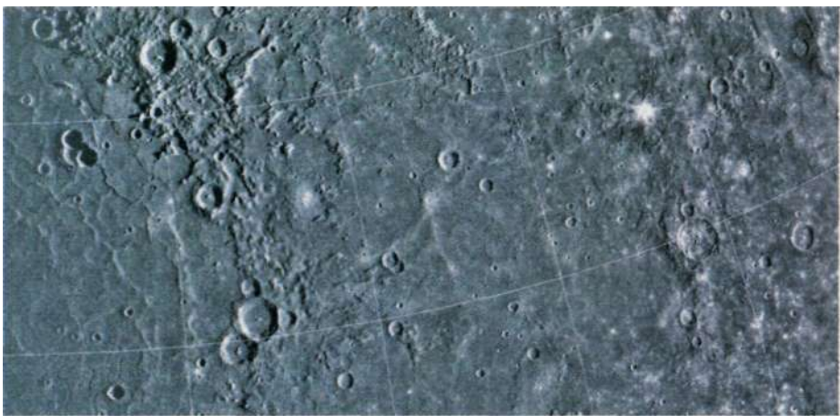
Рис. 8.3. Застывшая лава на равнине Калорис свидетельствует о том, что Меркурий 3 млрд лет назад был разогрет за счет внутреннего тепла, и тогда действовали сотни вулканов. Свежие кратеры образовались после падения метеоритов
