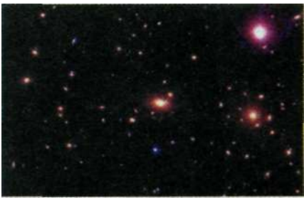
Рис. 15.7. Скопление галактик в созвездии Волосы Вероники
