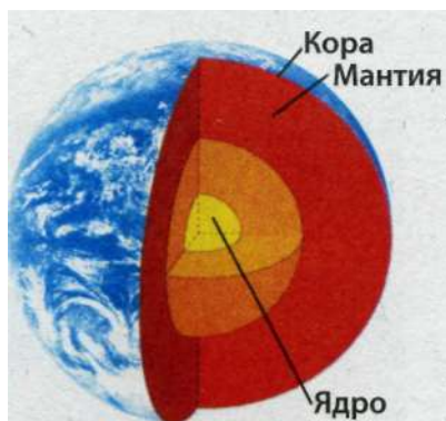
Рис. 7.4. Внутреннее строение Земли
