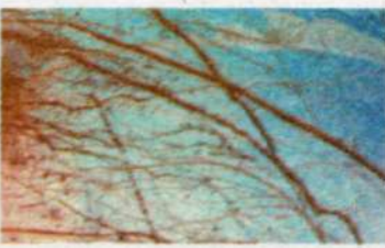
Рис. 10.4. Трещины в ледовом панцире Европы
