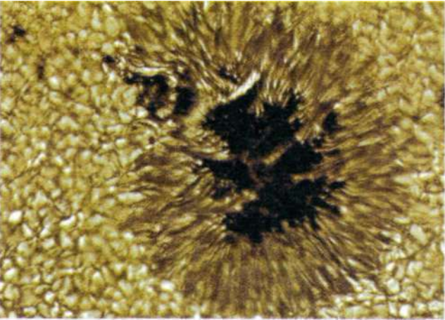
Рис. 12.5. Солнечное пятно
