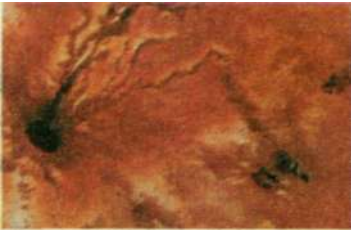
Рис. 10.3. На Ио много серы и действующих вулканов
