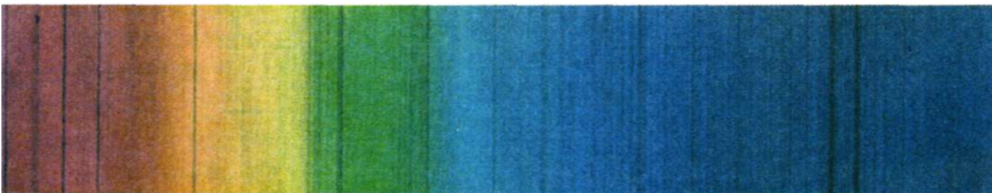
Рис. 12.4. Спектр Солнца. Темные линии поглощения образуются в хромосфере
