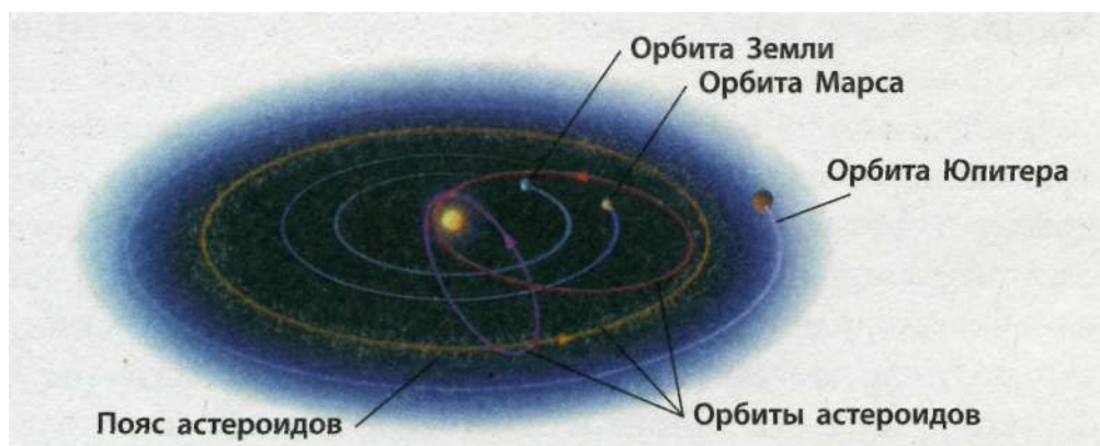
Рис. 11.3. Орбиты некоторых астероидов, пересекающих орбиту Земли
