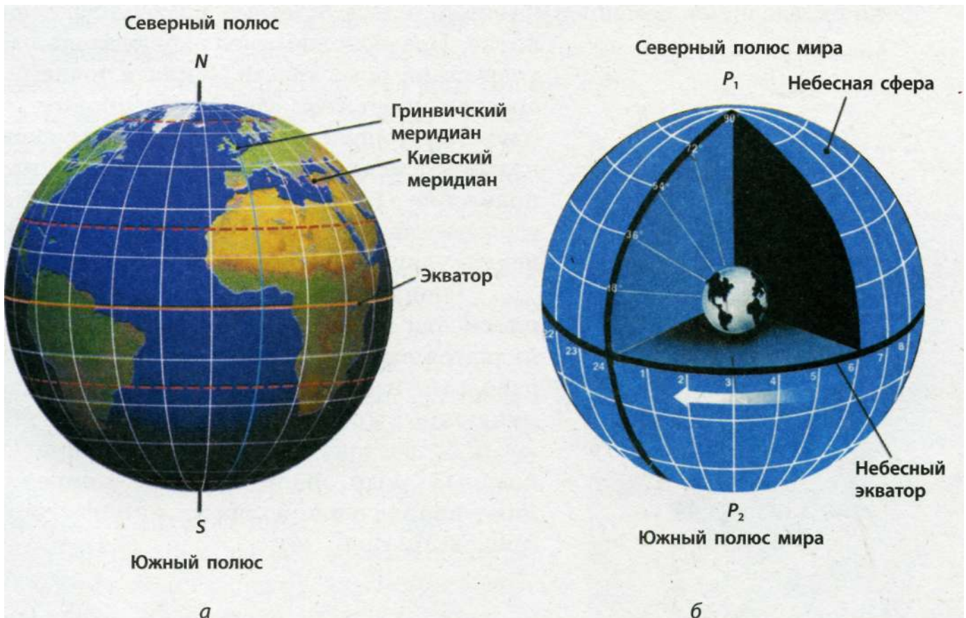
Рис. 2.3. Основные точки и линии системы координат: а — земной (географической), б — небесной
