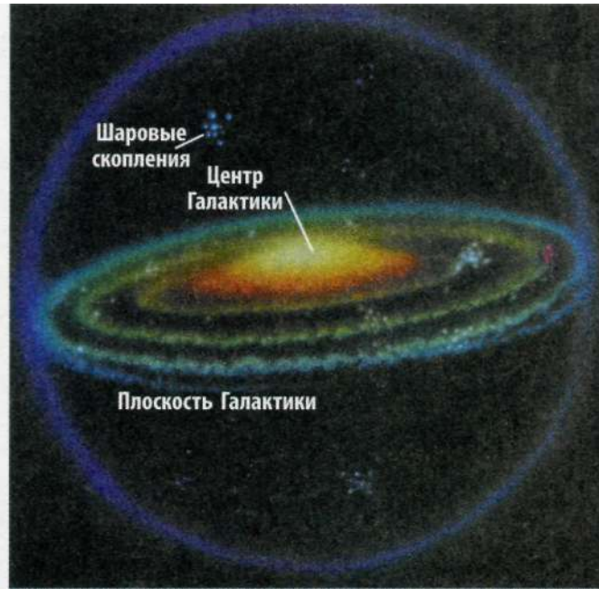
Рис. 15.3. Строение Галактики. В плоскости Галактики существуют газопылевые туманности, в которых рождаются молодые звезды и планетные системы
